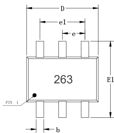
顶视图
