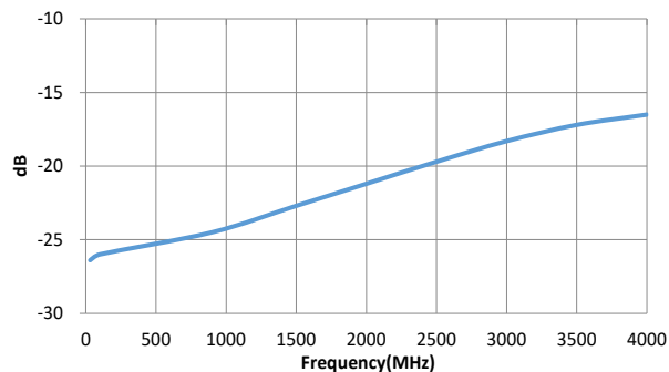
S12
