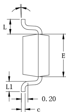
侧视图
