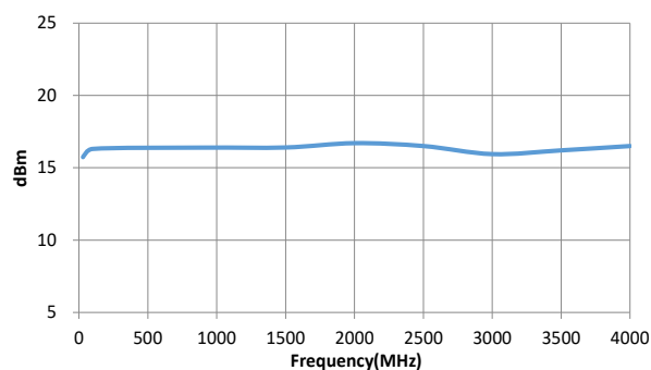
P1dB
