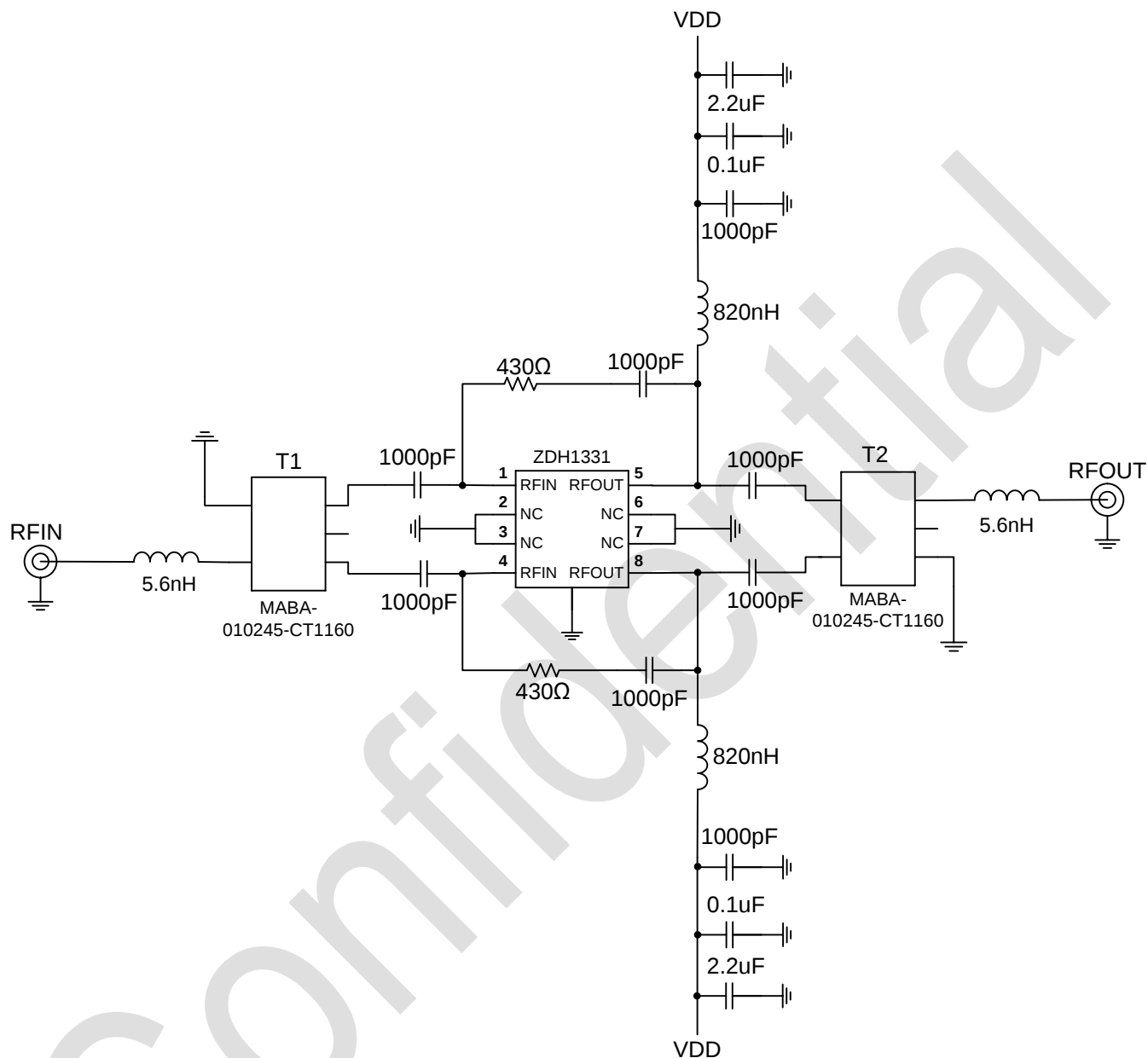
应用电路图（20MHz~1200MHz）
