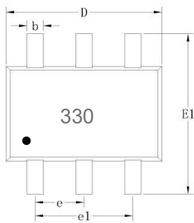
顶视图
