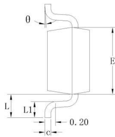
侧视图
