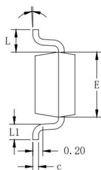
侧视图
