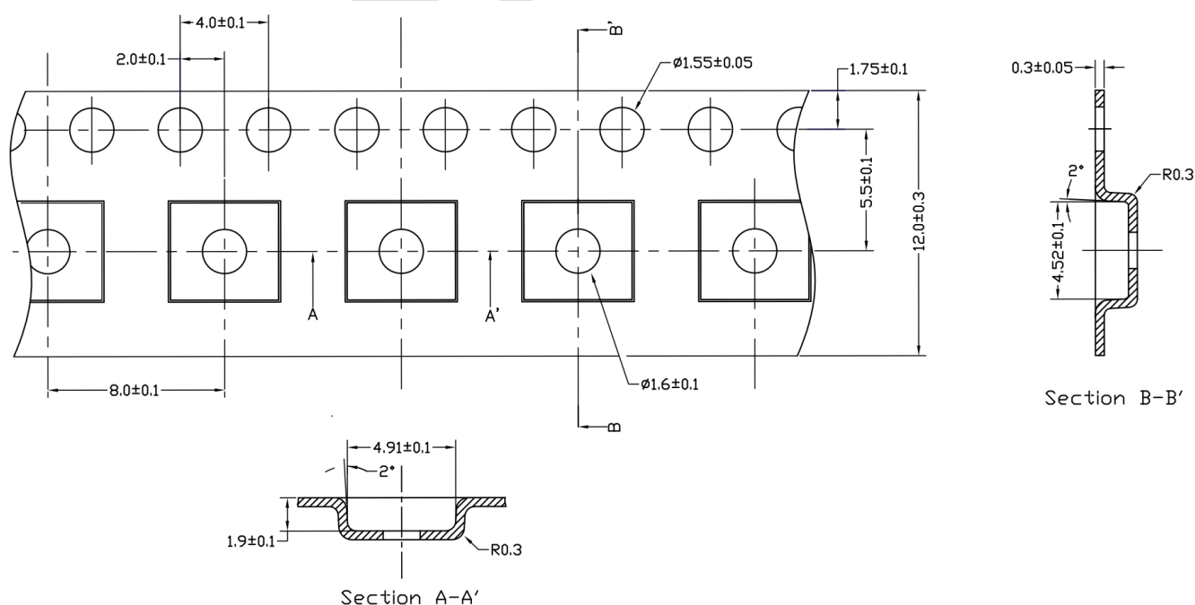
载带尺寸示意图
